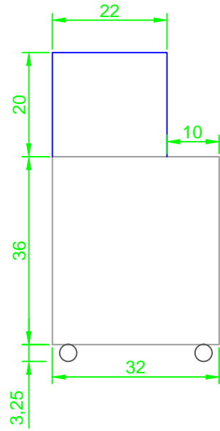
Side view Vue de côté
